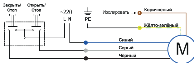
Схема подключения стационарной механической кнопки:
