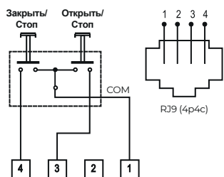
Схема подключения «сухих» контактов:
