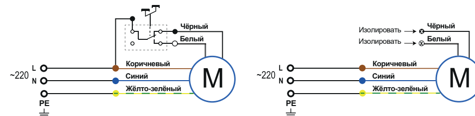
Универсальная схема подключения: Схема для управления радиопультом:
