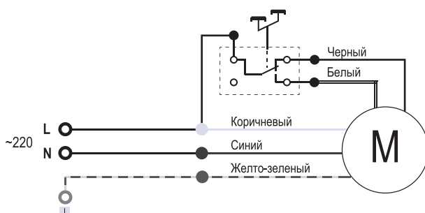
Подключение фазное + радио
