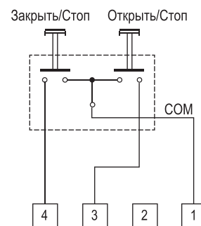
Схема для низковольтного управления электроприводом
